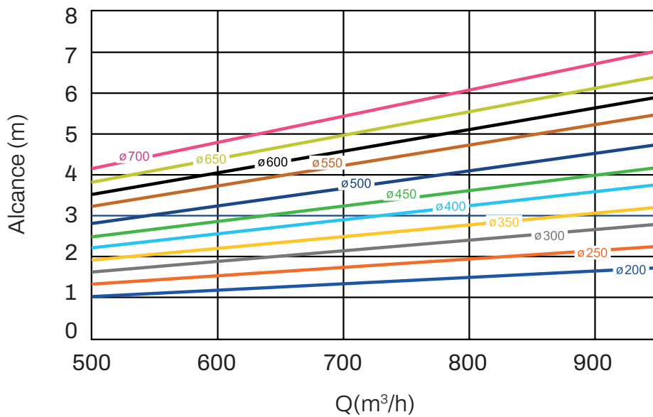
E-LO/CA 700 x 150
